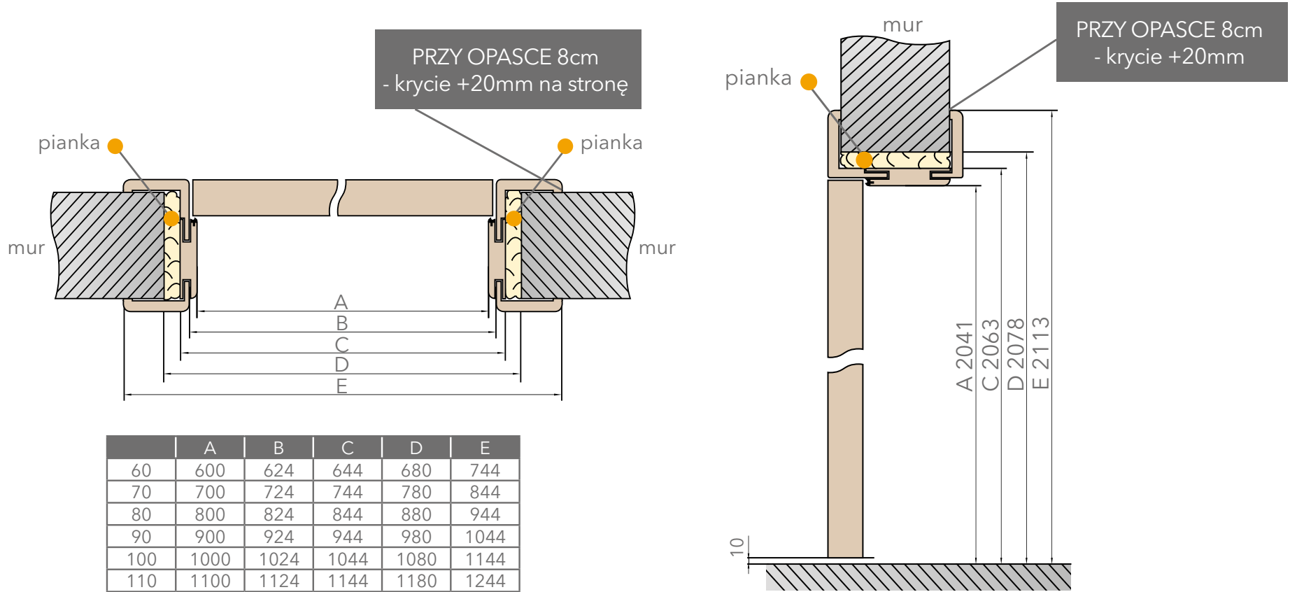
SCHEMAT DRZWI BEZPRZYLGOWYCH W OŚCIEŻNICY REGULOWANEJ
