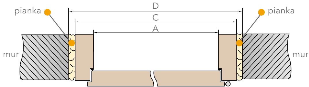
SCHEMAT DRZWI PRZYLGOWYCH W FUTRYNIE STAŁEJ
