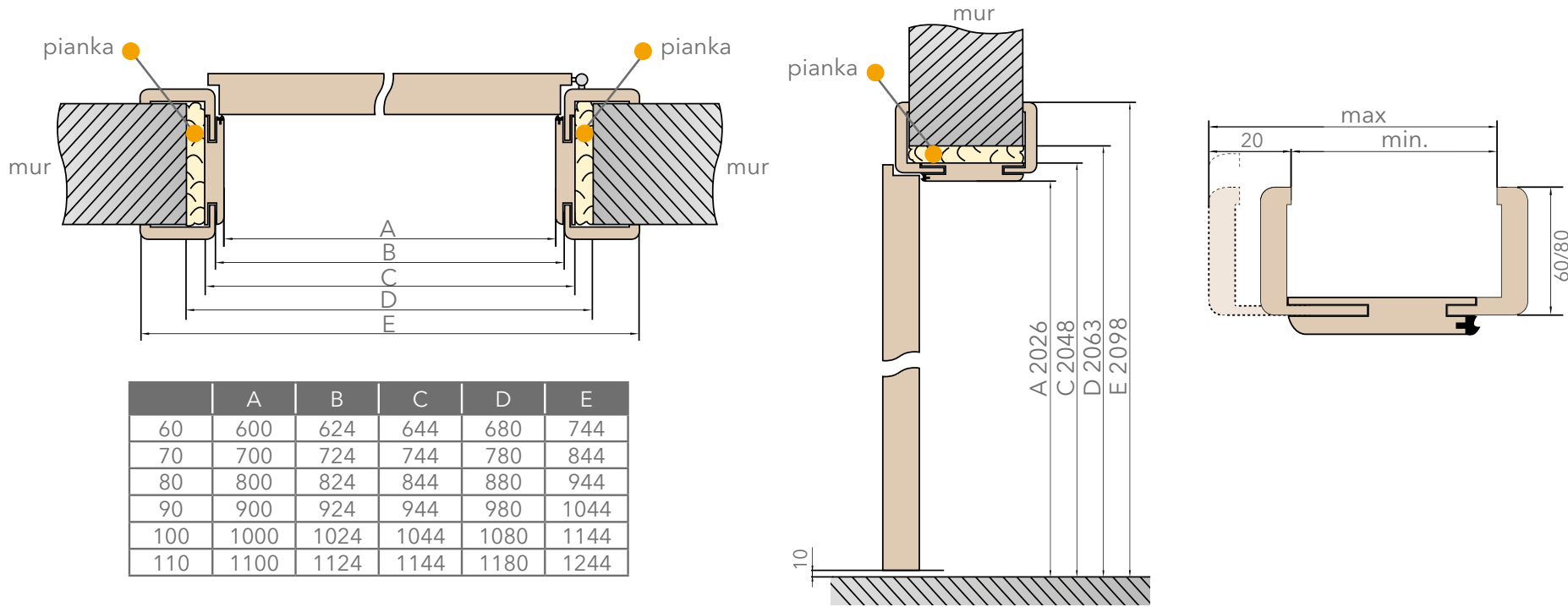
SCHEMAT DRZWI PRZYLGOWYCH W OŚCIEŻNICY REGULOWANEJ
